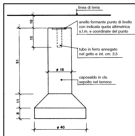
FIG. 3 - Tipo di caposaldo
